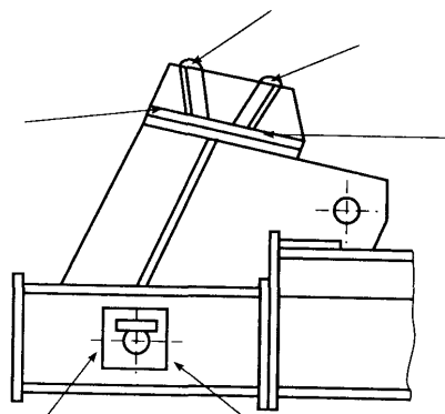
Узел крепления опоры к ходовой тележке козлового крана ККС-10.
